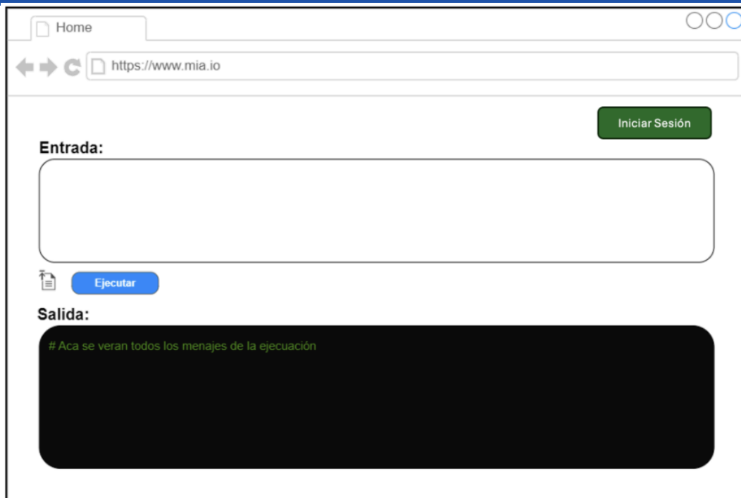
Figura 2 - Página Principal
